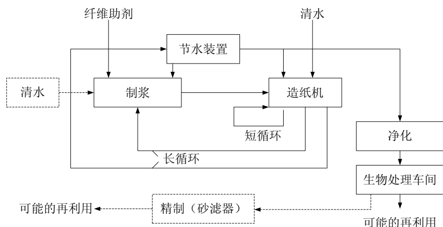
图5 水回路的优化设计
